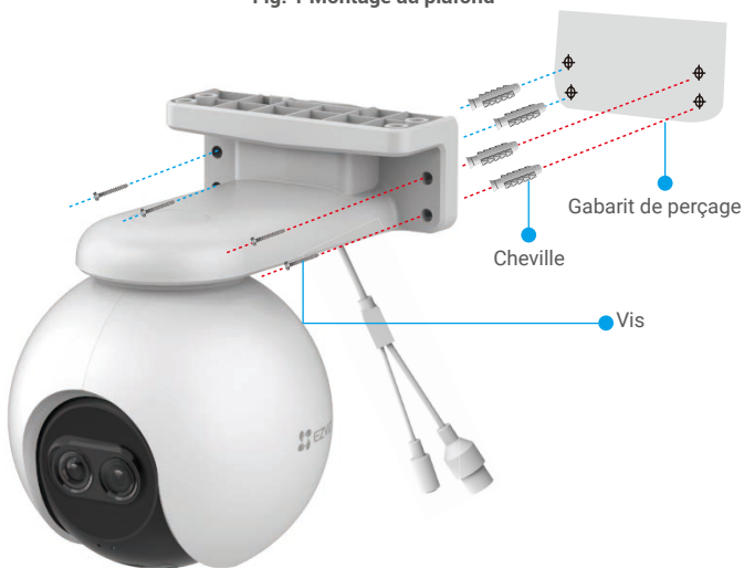
Fig. 2 Montage mural
